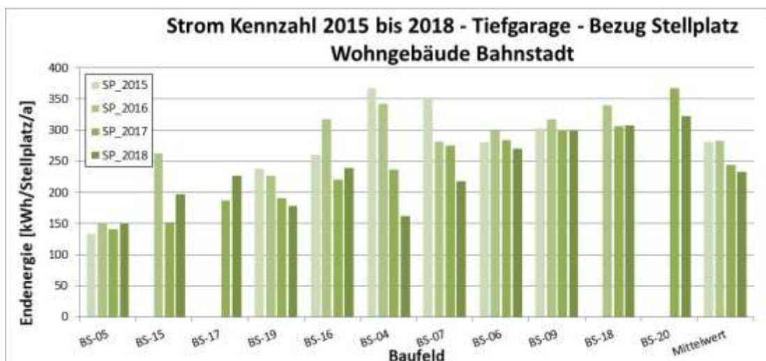
Abbildung 19: Strom Tiefgarage, Bezug Stellplatz
