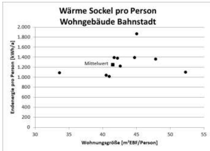
Abbildung 7: Wärme 2018 personenbezogen
