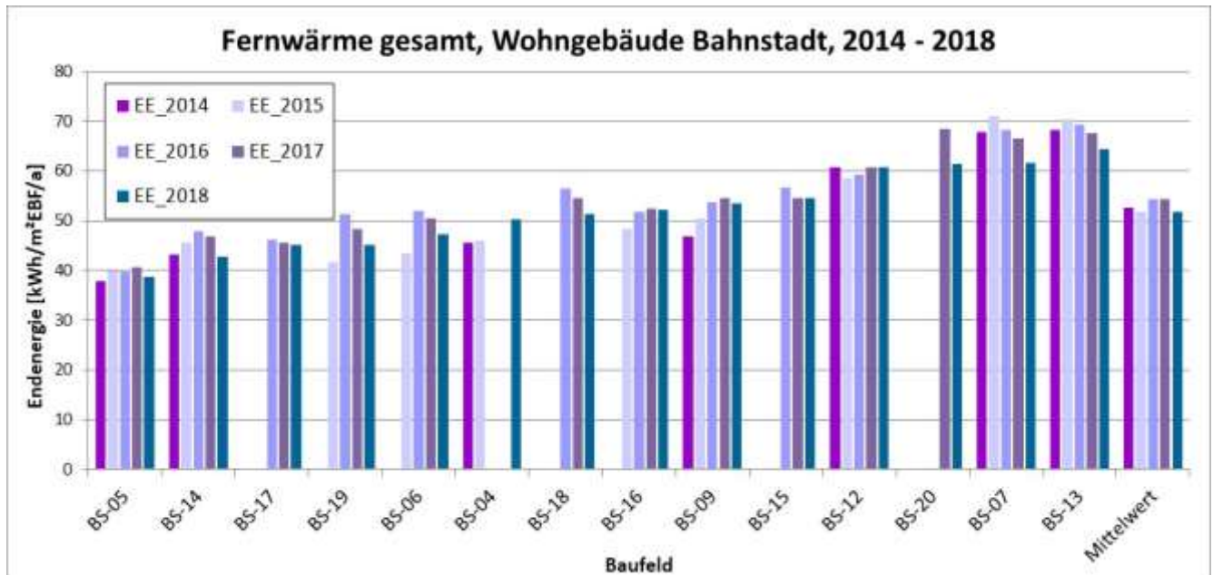
Abbildung 1: Fernwärme gesamt
