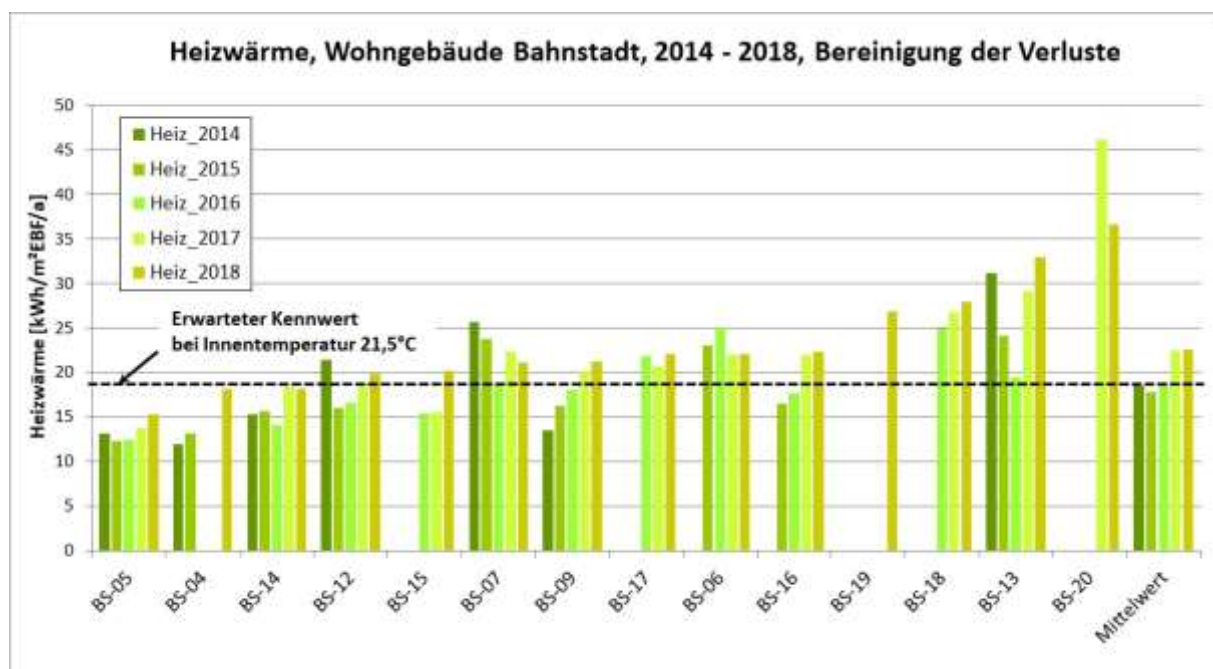
Abbildung 5: Heizwärme der Wohnbaufelder, Verluste witterungsbereinigt, Messabweichung \pm 4 kWh/(m 2 a)
