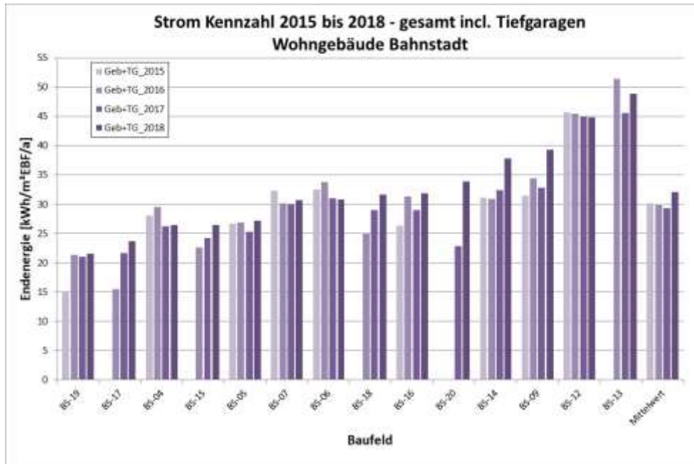
Abbildung 12: Strom gesamt incl. Tiefgaragen
