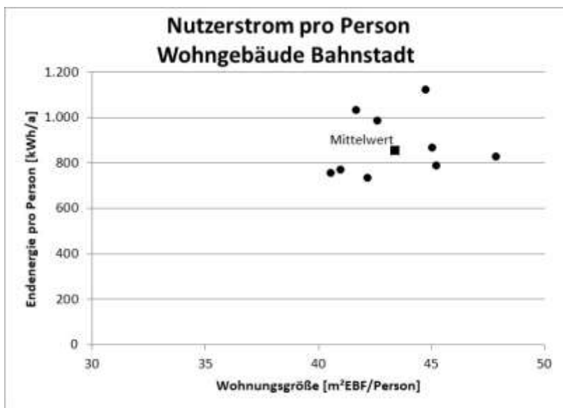
Abbildung 17: Strom 2018 personenbezogen
