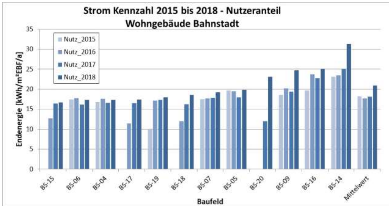
Abbildung 15: Strom Nutzer
