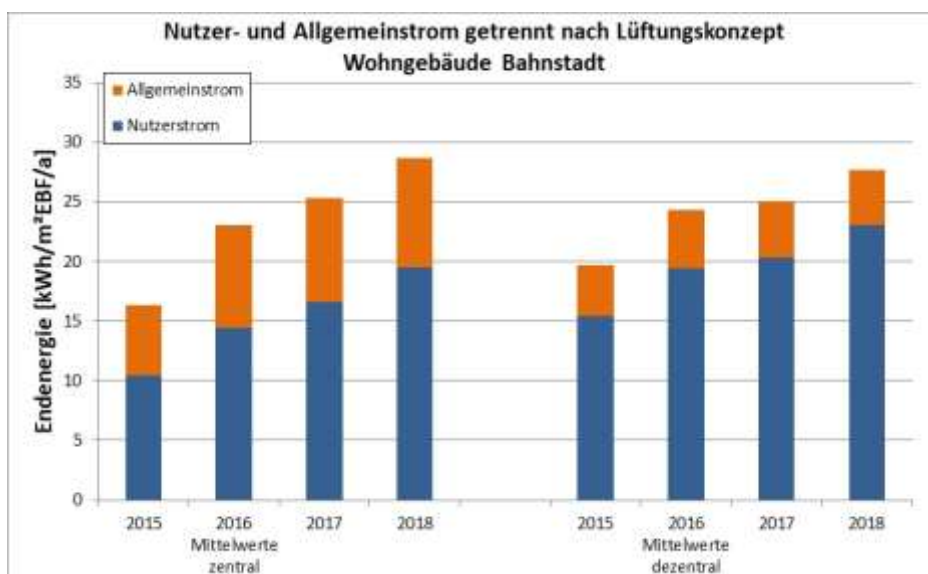
Abbildung 16: Mittelwerte der Baufelder mit zentralem / dezentralem Lüftungskonzept
