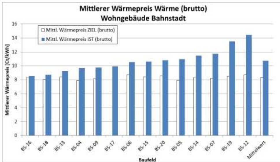
Abbildung 11: Mittlerer Wärmepreis, Bezugsjahr 2018
