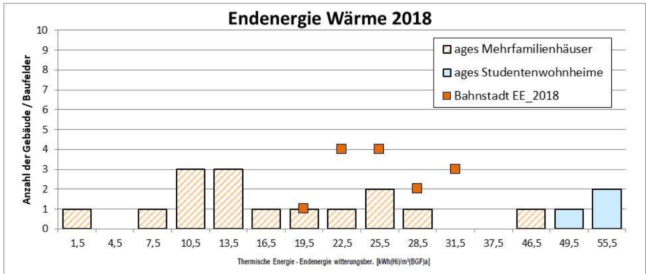
Abbildung 8: Wärmeverbrauch – Häufigkeitsverteilung (in Anlehnung an [ages 2015], Grafik 22)
