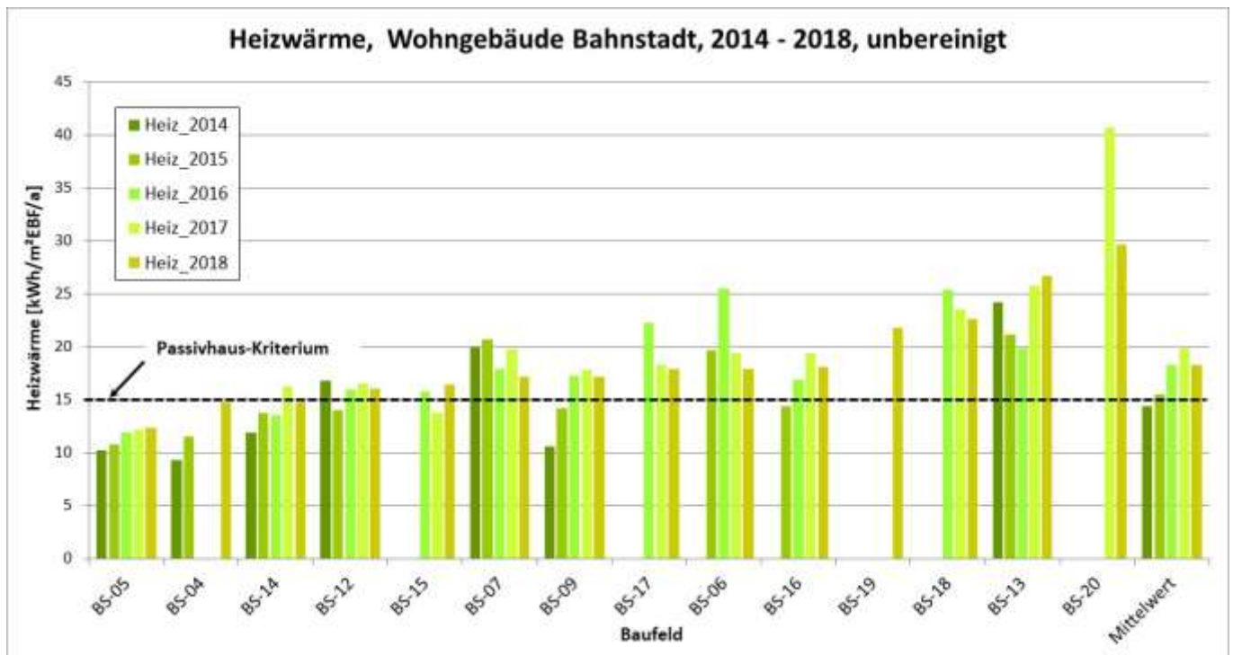
Abbildung 3: Heizwärme der Wohnbaufelder, unbereinigt, Messabweichung im Bereich \pm 4 \text{ kWh}/(\text{m}^2\text{a})
