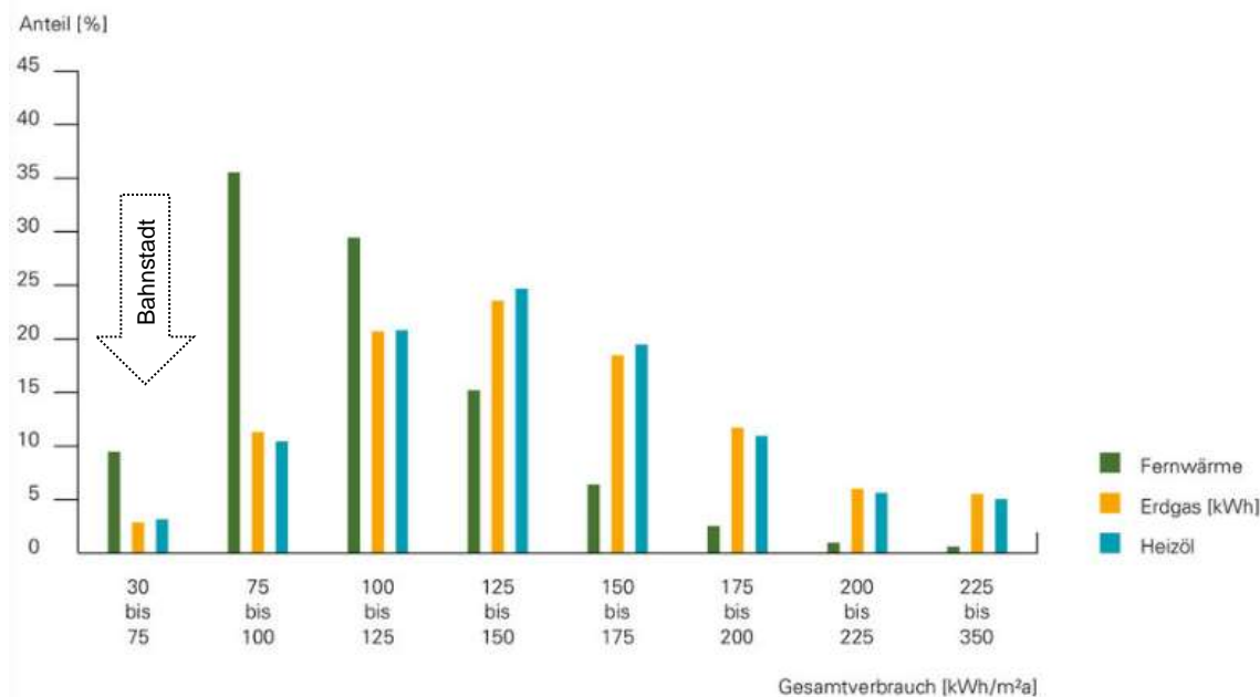
Abbildung 10: Häufigkeitsverteilung des spezifischen Gesamtverbrauchs in verbundenen Anlagen im Bundesdurchschnitt, Bezug auf Wohnfläche (aus [Techem 2018], nicht witterungsbereinigt)
