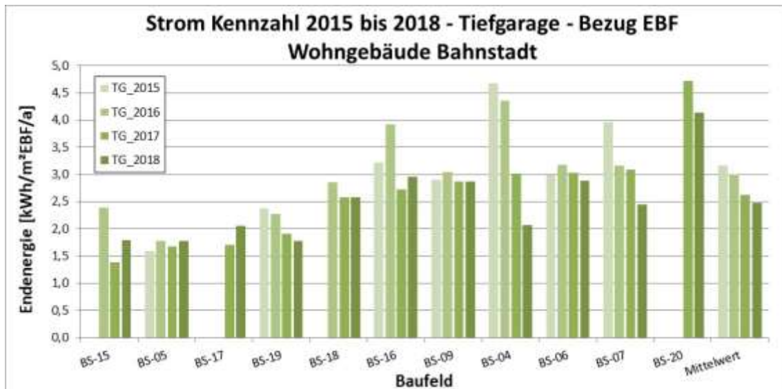
Abbildung 18: Strom Tiefgarage, Bezug EBF
