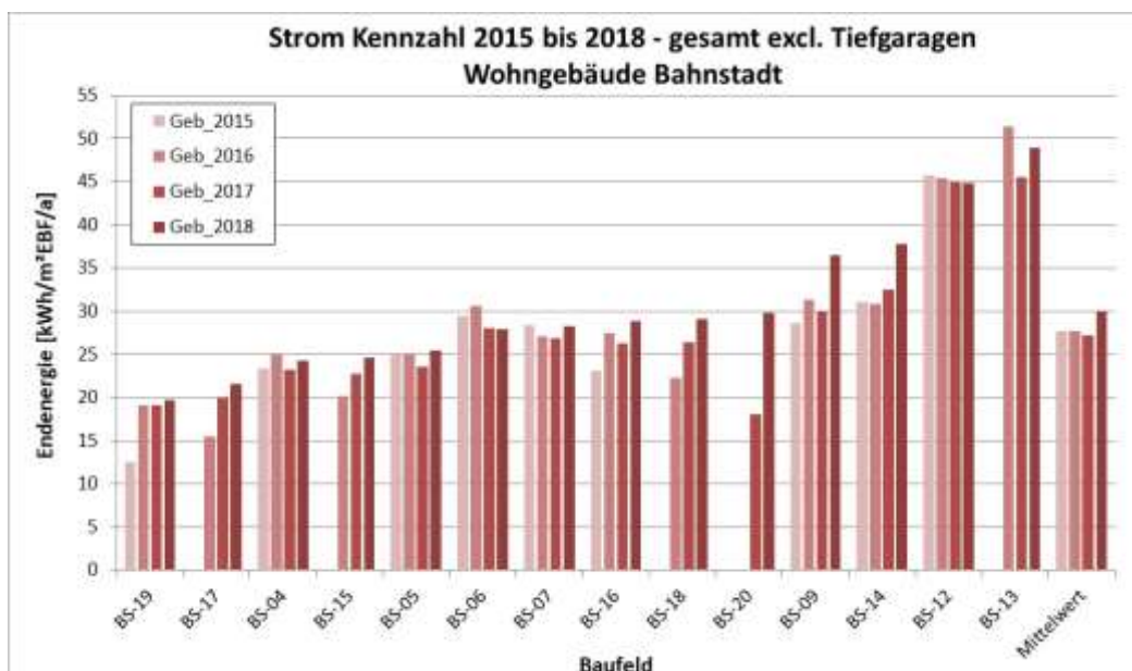
Abbildung 13: Strom gesamt excl. Tiefgaragen
