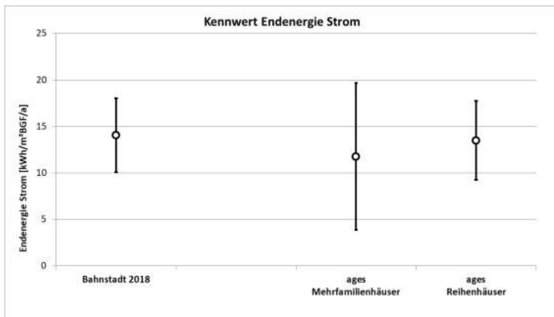
Abbildung 21: Kennwert Endenergie Strom – Mittelwert und Standardabweichung
