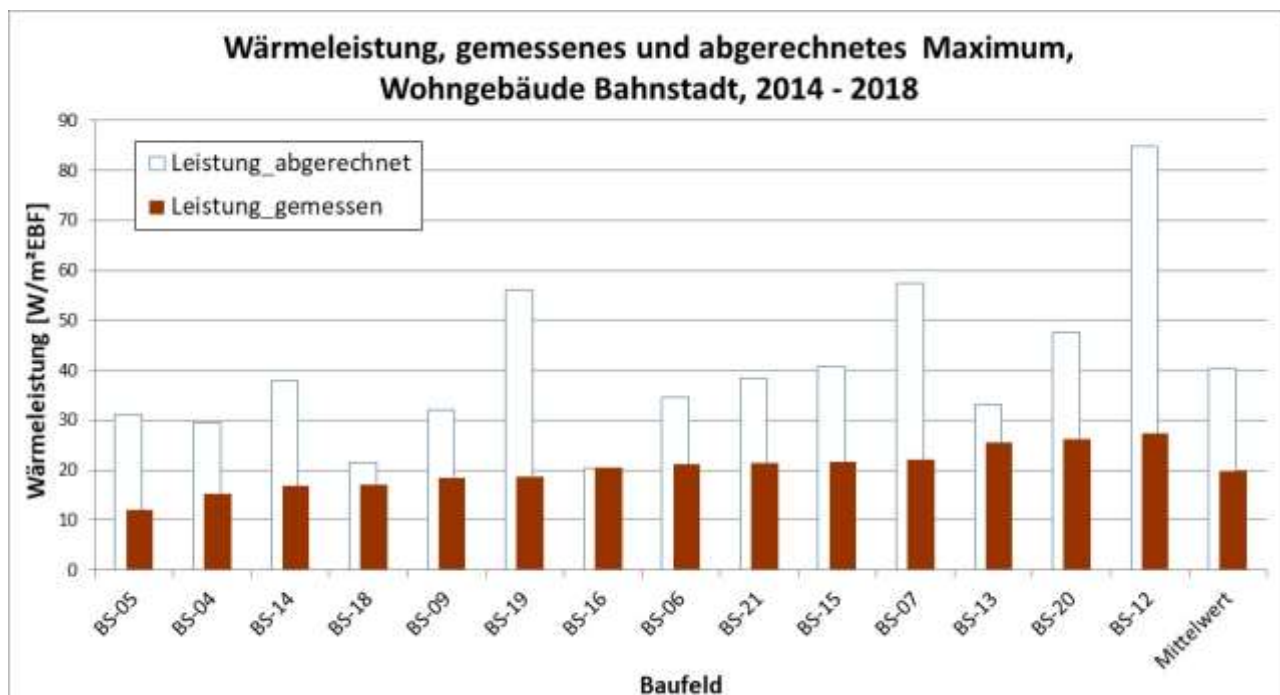
Abbildung 6: Leistungsbezug
