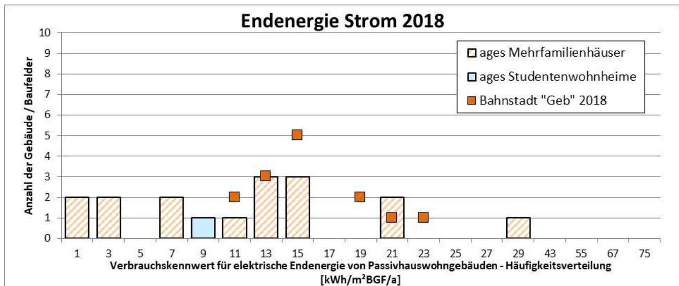
Abbildung 20: Stromverbrauch – Häufigkeitsverteilung (in Anlehnung an [ages 2015], Grafik 20)
