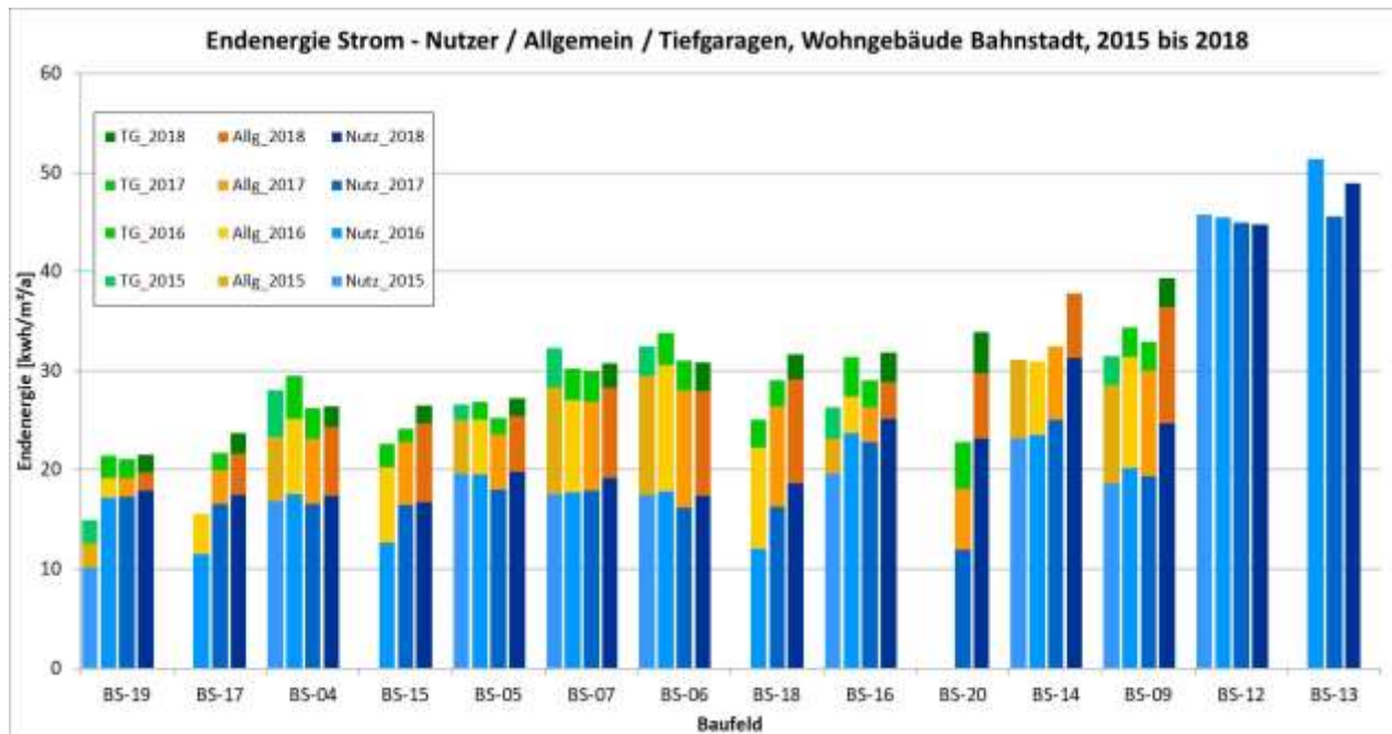
Abbildung 14: Strom gesamt - aufgetrennt
